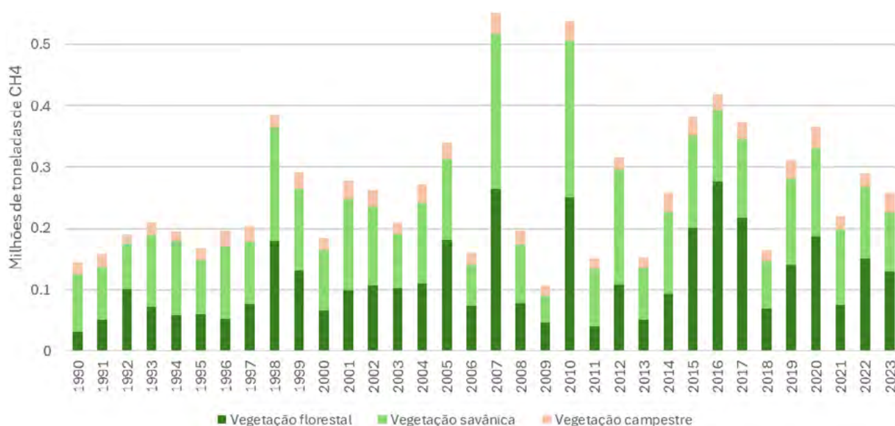
Figura 4.3.2.b. Histórico das emissões de metano ( \text{CH}_4 ) por queimadas por tipo de vegetação no Brasil. Fonte: SEEG Coleção 12 (2024)
