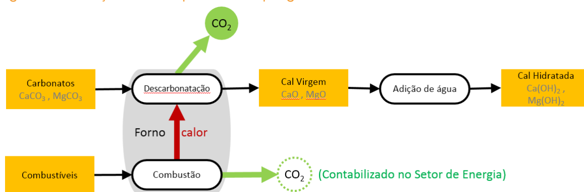
Figura 5: Produção de cal e processos que geram emissões
