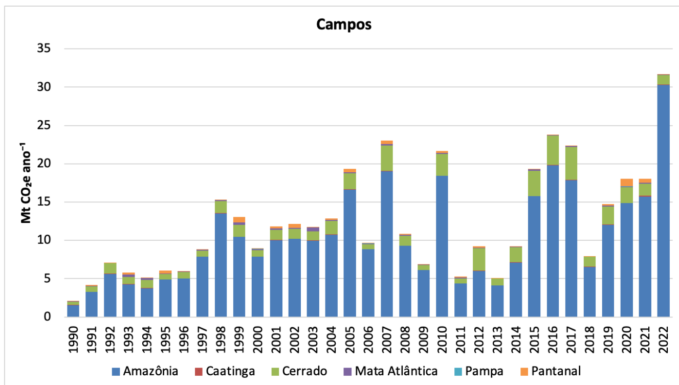
Figura 7. Emissões líquidas de CO 2 e (GWP AR5) por fogo em áreas naturais de florestas, savanas e campos não associadas a desmatamento.
