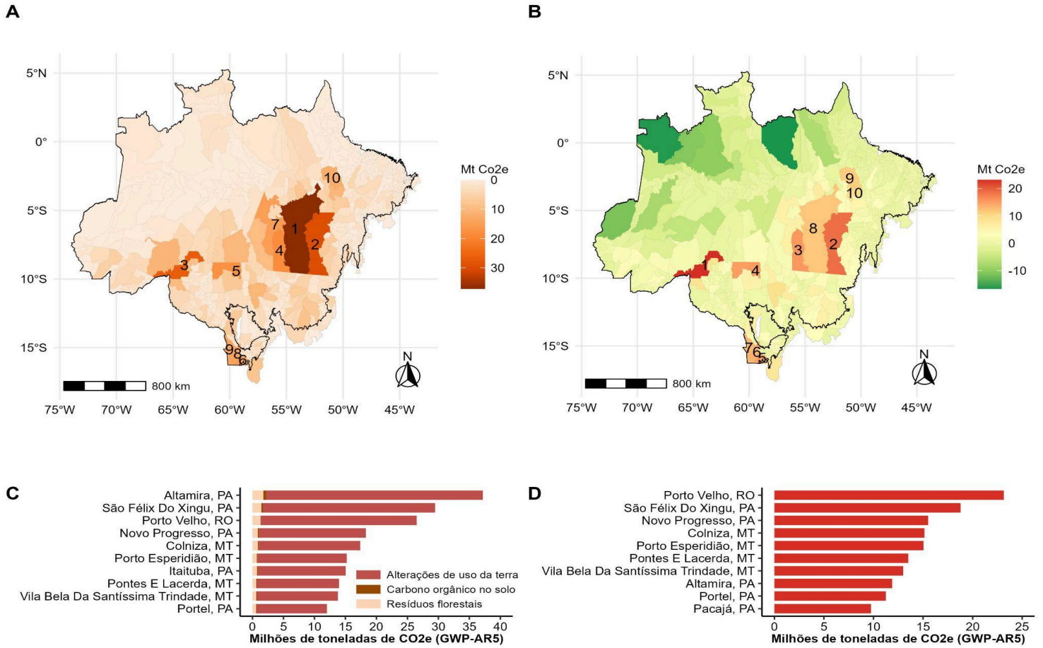
Figura 14. Localização e ranking dos dez municípios no bioma Amazônia que mais emitem em 2022, em termos de emissões brutas (A e C) e emissões líquidas (B e D).
