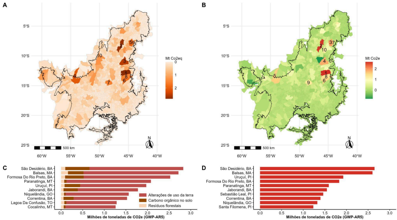
Figura 16. Localização e ranking dos dez municípios no bioma Cerrado que mais emitem em 2022, em termos de emissões brutas (A e C) e emissões líquidas (B e D)
