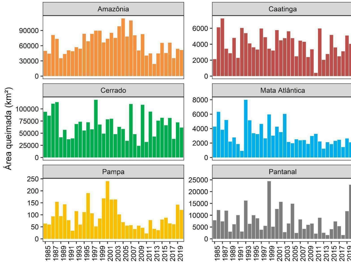
Figura 3. Distribuição temporal (1985-2020) da área queimada (km 2 ) nos seis biomas brasileiros. Fonte: MapBiomias Fogo.
