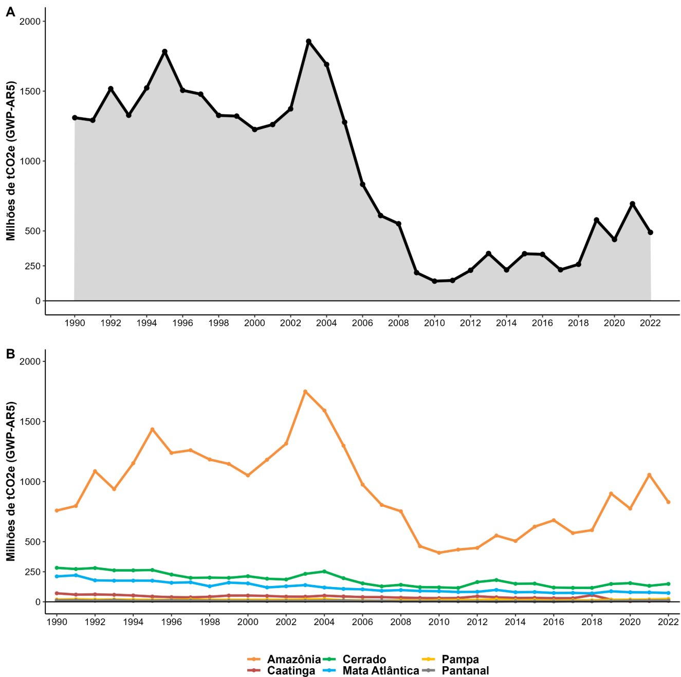
Figura 11. Emissões líquidas totais nacionais (a) e Emissões brutas por bioma (b) em milhões de toneladas de CO 2 e (GWP AR5) associadas ao setor MUT ao longo do período de 1990-2022.
