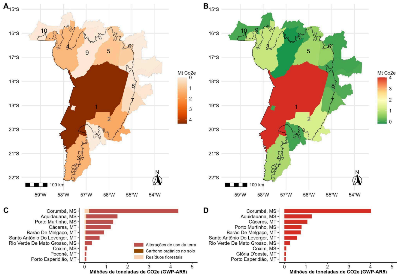
Figura 19. Localização e ranking dos dez municípios no bioma Pantanal que mais emitem em 2022, em termos de emissões brutas (A e C) e emissões líquidas (B e D).
