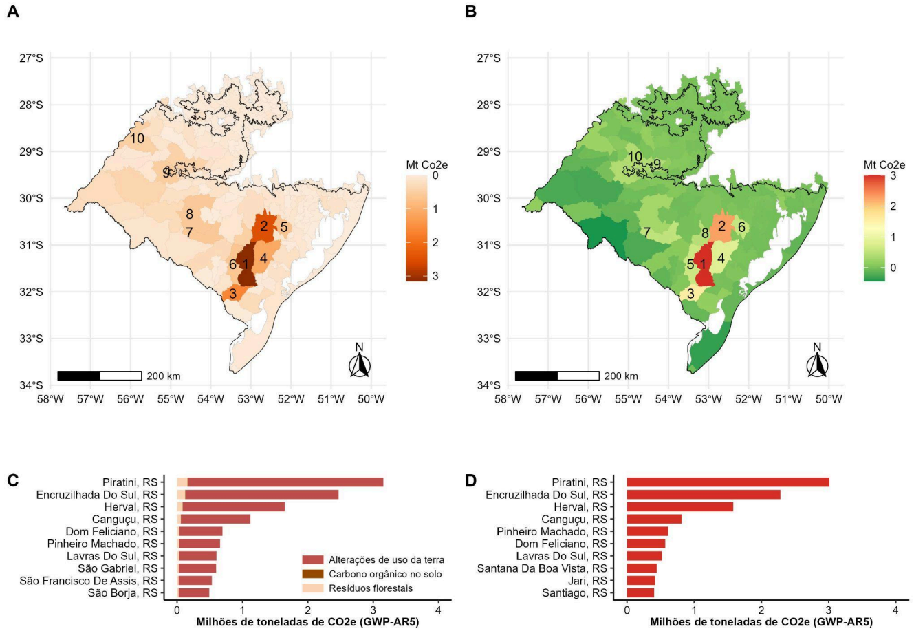
Figura 18. Localização e ranking dos dez municípios no bioma Pampa que mais emitem em 2022, em termos de emissões brutas (A e C) e emissões líquidas (B e D).
