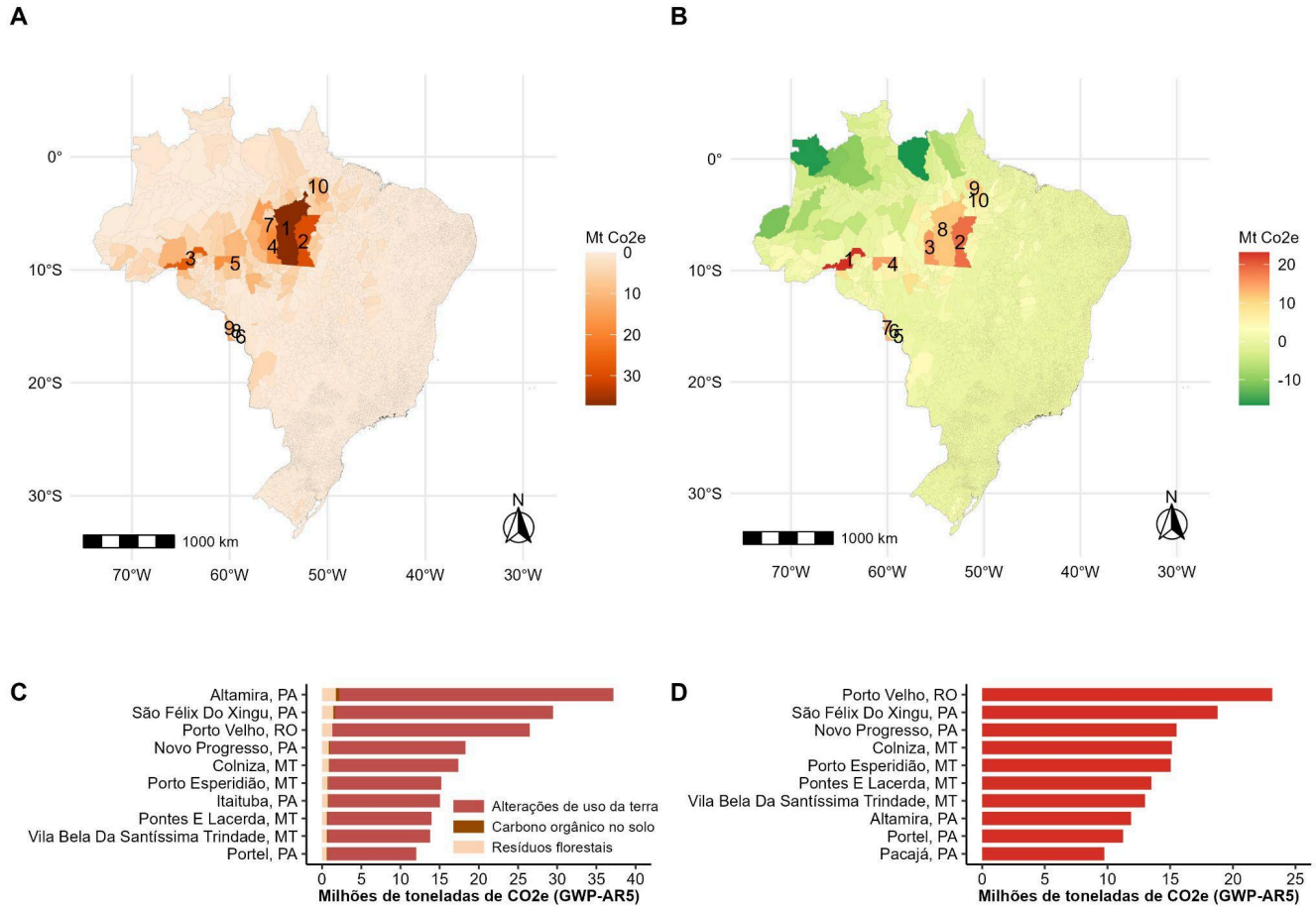
Figura 13. Localização e ranking dos dez municípios brasileiros que mais emitem em 2022, em termos de emissões brutas (A e C) e emissões líquidas (B e D).
