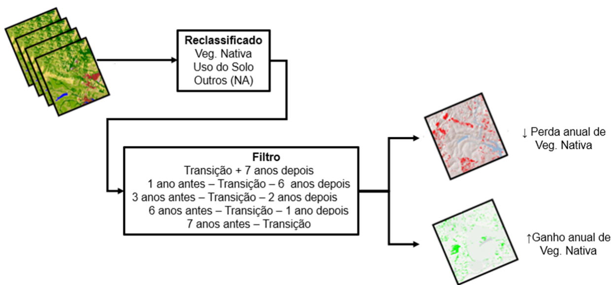
Figura 3. Regras da janela temporal para a geração das máscaras de perda (desmatamento) e ganho (regeneração) de vegetação nativa a cada ano.
