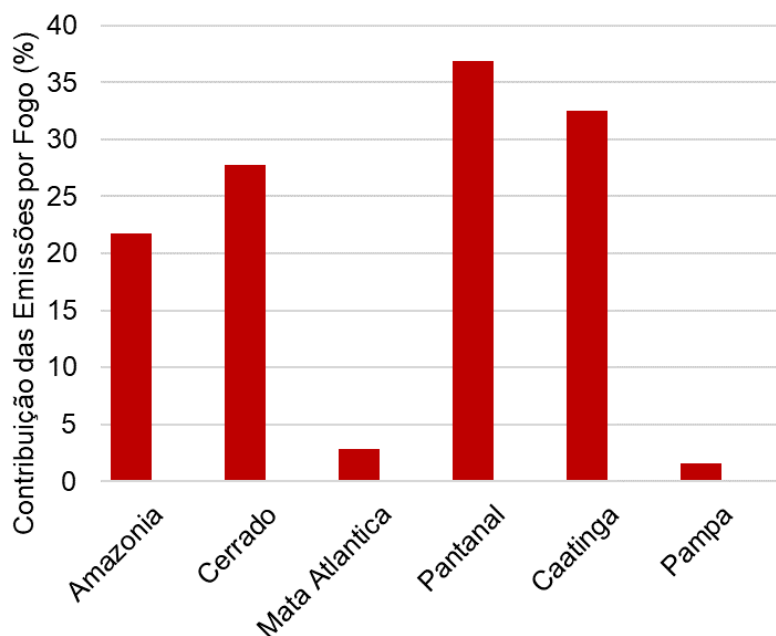
Figura 8. Contribuição percentual das emissões líquidas de CO 2 e (GWP AR5) por fogo não associado a desmatamento quando essas são adicionadas às emissões do setor MUT. Os valores percentuais representam a média da contribuição entre 1990-2022.
