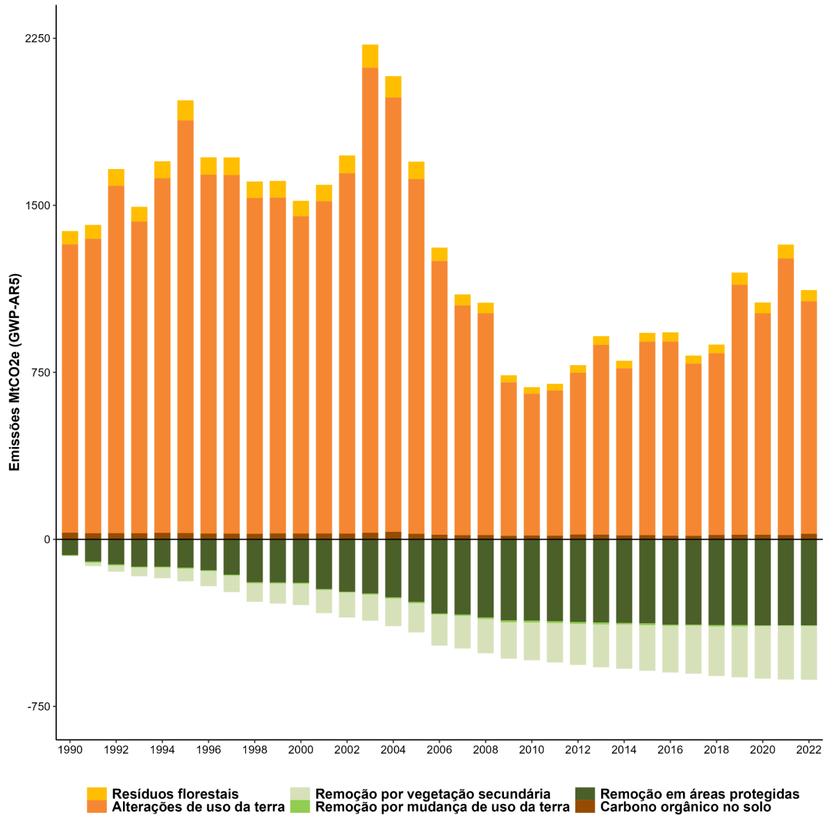
Figura 10. Emissões brutas totais nacionais em milhões de toneladas de CO 2 e (GWP AR5) por categoria do setor MUT ao longo do período de 1990-2022.
