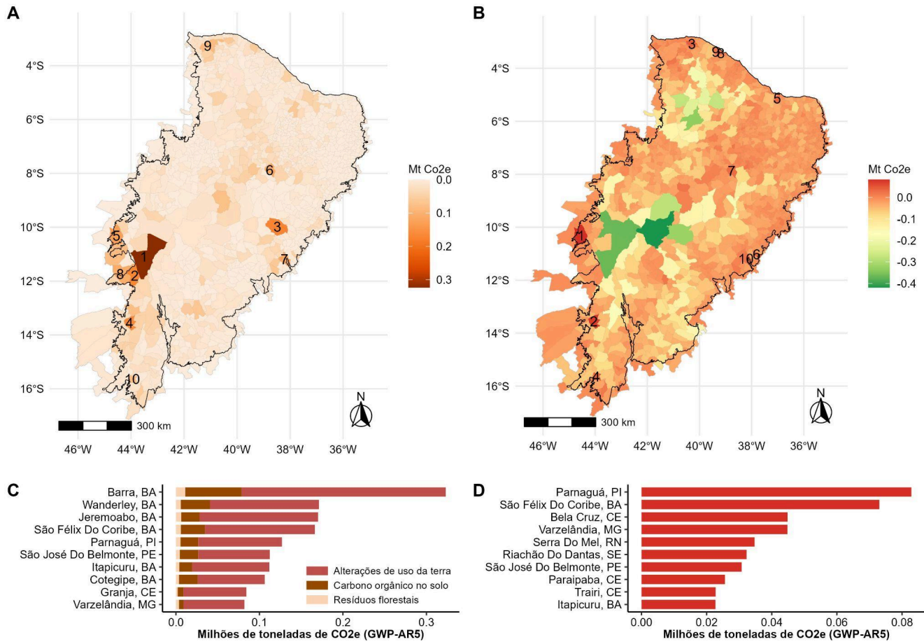
Figura 14. Localização e ranking dos dez municípios no bioma Caatinga que mais emitem em 2022, em termos de emissões brutas (A e C) e emissões líquidas (B e D).
