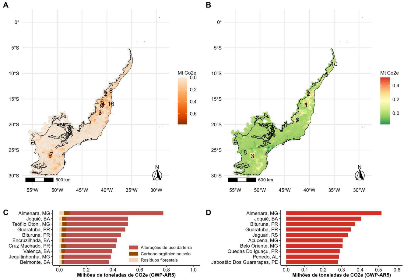
Figura 17. Ranking e localização dos dez municípios no bioma Mata Atlântica que mais emitem em 2022, em termos de emissões brutas e emissões líquidas.
