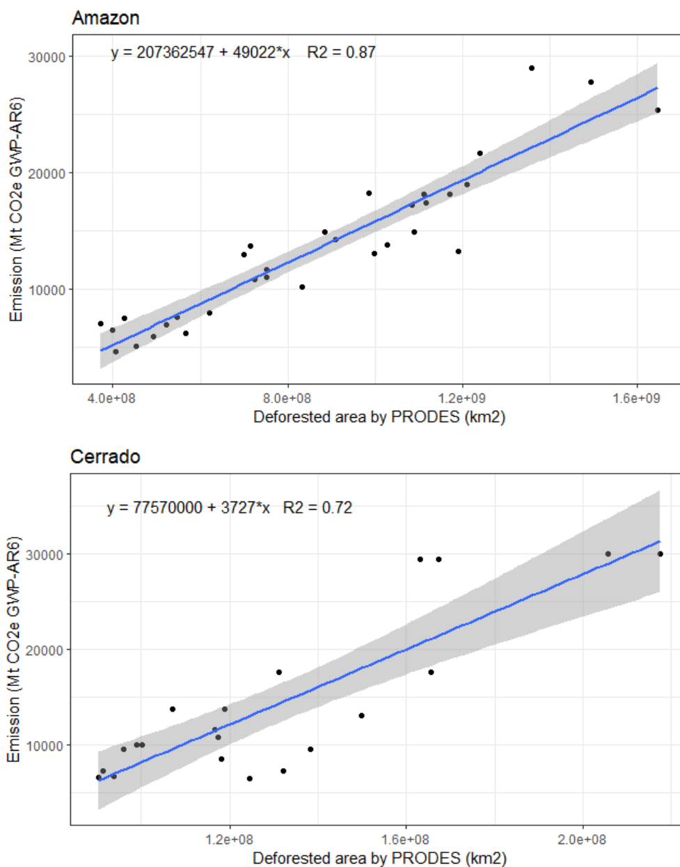
Figura 5. Regressões lineares das emissões do SEEG 11 em relação à taxa de desmatamento oficial (Prodes) nos biomas Amazônia e Cerrado utilizadas para estimar as emissões no último ano, 2022.
