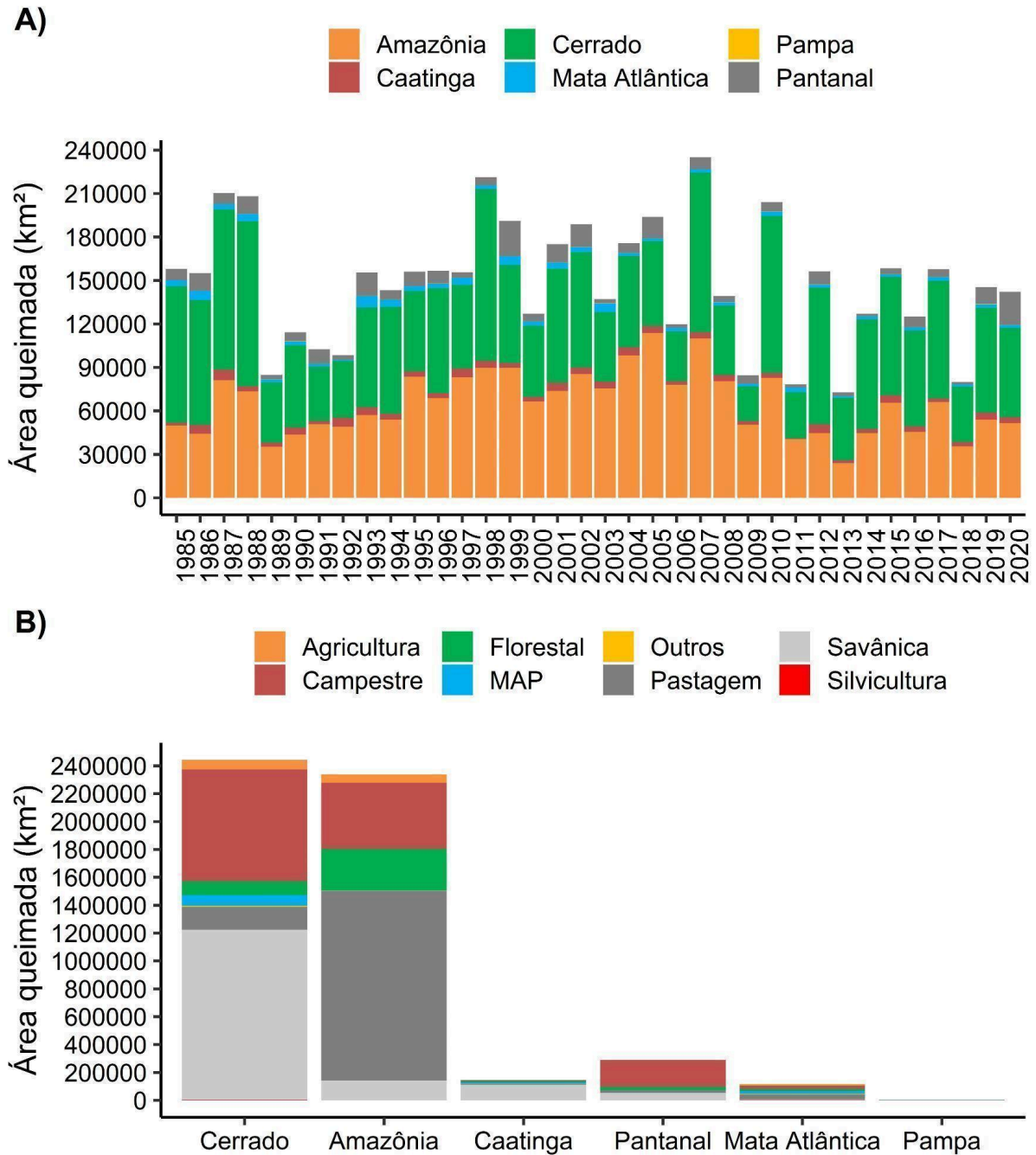
Figura 2. Distribuição temporal (1985-2020) da área queimada ( \text{km}^2 ) nos seis biomas brasileiros (A) e em suas principais coberturas e usos da terra (B). MAP = Mosaico de Agricultura e Pastagem. Fonte: MapBiomas Fogo.
