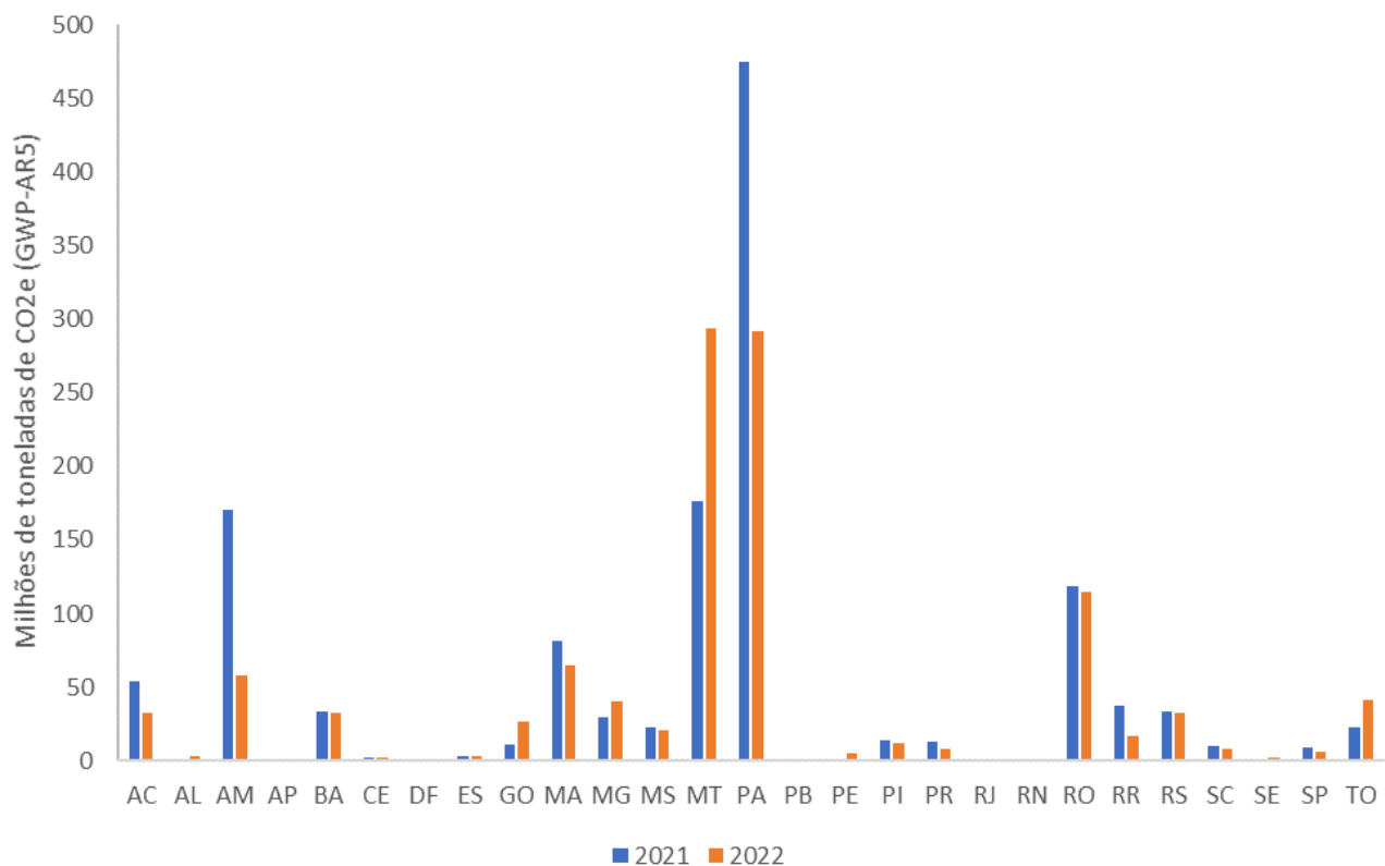
Figura 12. Emissões brutas por estado em milhões de toneladas de CO 2 e (GWP AR5) associadas ao setor MUT em 2021 e 2022.
